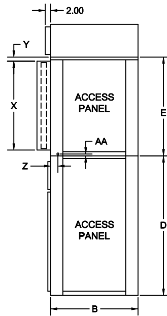
LH SIDE
