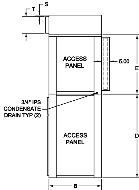
LH SIDE
