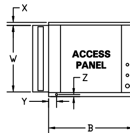
LH SIDE
