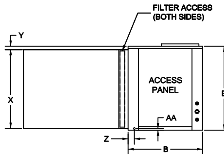
LH SIDE
